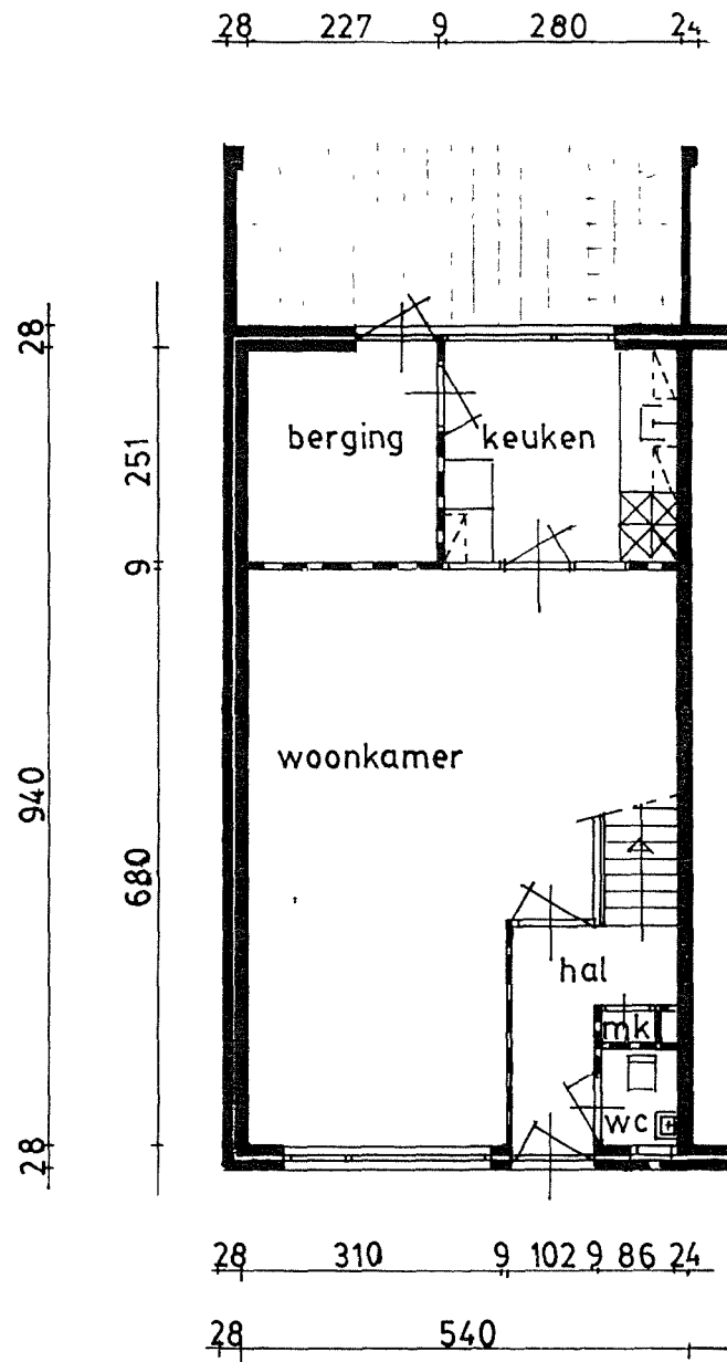
BEGANE GROND
